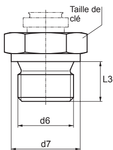
Filetages cylindriques
