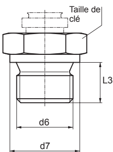
Filetages cylindriques
